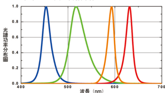
R/G/B LED典型发射光谱
