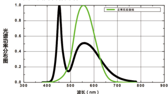
典型白光发射光谱
